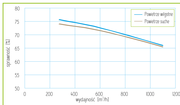
Charakterystykę sprawności podano dla parametrów: SWNM**.
